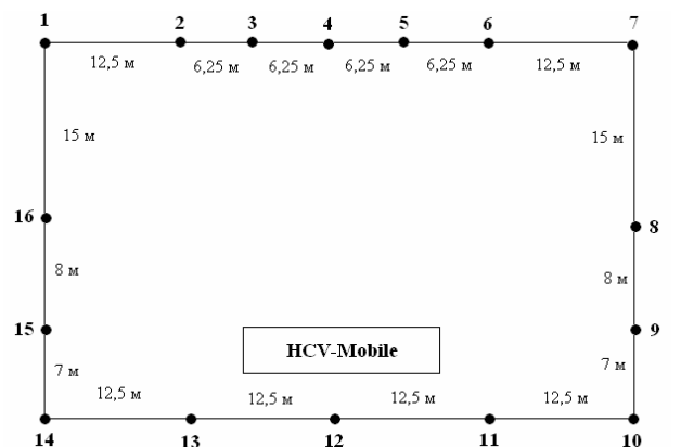
Рис. 4.1. Схема расположения точек измерения при проведении измерений максимальной дозы тормозного излучения на границе зоны ограничения доступа мобильного комплекса 2-го типа за одно сканирование.
