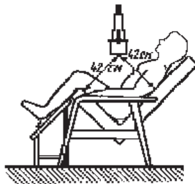
Рис. 5.2. Геометрия измерения «стандартное кресло»
