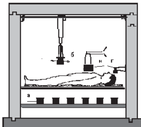
Рис. 5.1. СИЧ экспертного класса, геометрия измерения «лежа»
