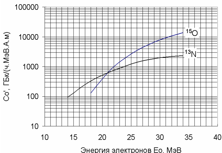
Рис. 1. Зависимость постоянной скорости образования ( C'_0 ) радионуклидов 13 N и 15 O от энергии электронов (вольфрамовая мишень)
